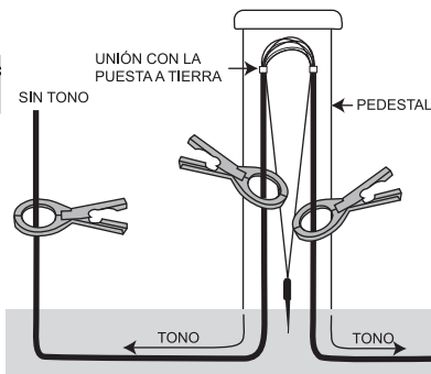
Fig. 10. Puntos de acoplamiento
