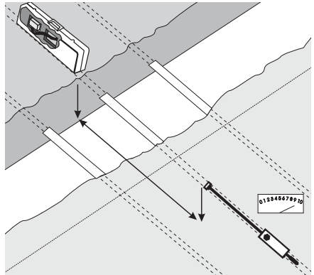
Fig. 16. Ubicación de la antena directamente arriba de un servicio público
