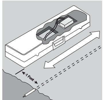
Fig. 14. Ubicación de la antena
