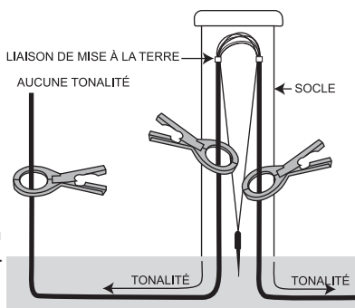
Fig. 10. Points de couplage
