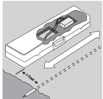
Fig. 14. Positionnement de l'antenne
